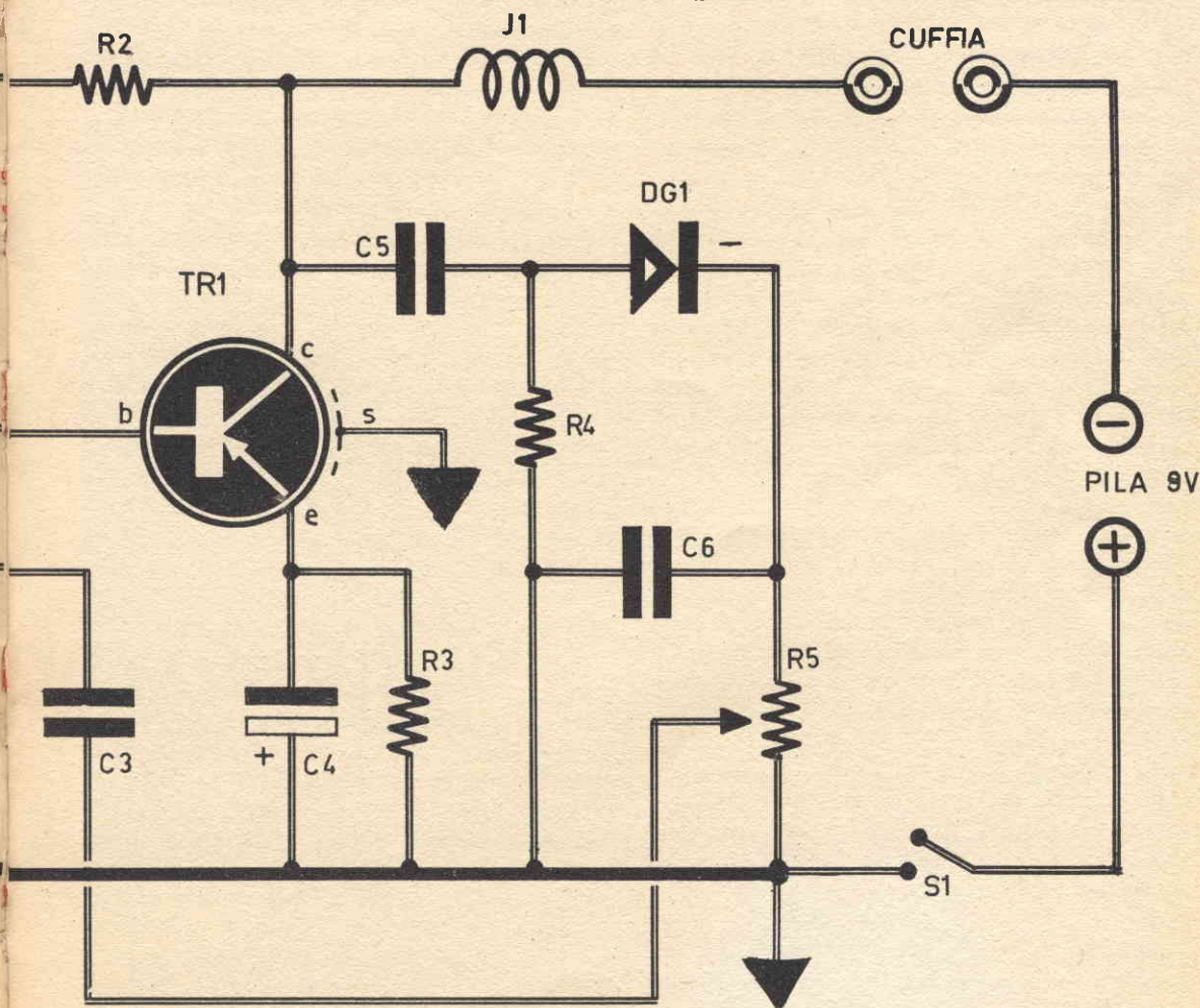
FIG. 1 - Schema teorico della prima versione del ricevitore descritto nel testo
